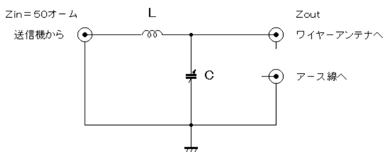
L型マッチング回路 CYTEC 2013/07
