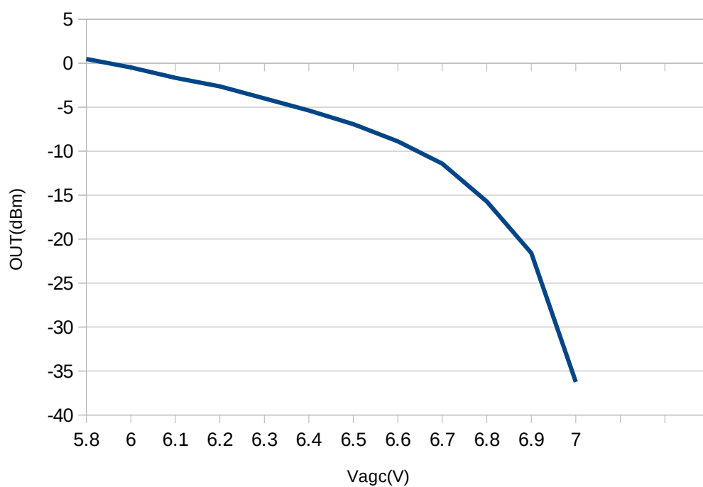
CY7045 AGC特性
